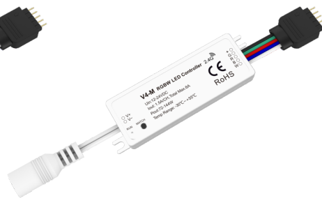
V4-M(DJ) Verze DC konektor samice vstup / 5P konektor samice výstup
